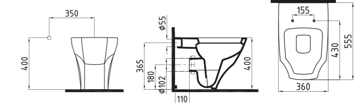
ELITE BTW WC PAN 56 cm FRKK05601VPOW3QA0 560x360 mm
