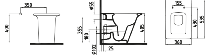
ARTOS BTW WC PAN 54 cm LTKK05401VPOW3QA0 540x360 mm
