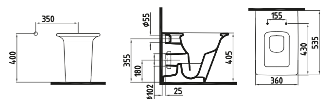
ARTOS BTW WC PAN 54 cm LTKK05401VPOW3QA0 540x360 mm
